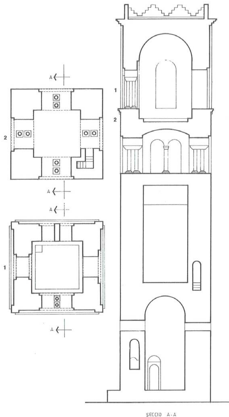
Campanar de Sant Pere de Vilamajor. Secció longitudinal i seccions transversals de les dues plantes superiors (planimetria: M. Anglada)
