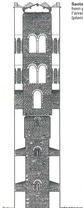
Campanar de l'església de Santa Maria de Seva (Osona). Segle XII. Extret de la Catalunya romànica .
