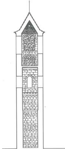
Església i campanar de Sant Julià Sassorba (Gurb, Osona). Segona meitat segle XI. Extret de la Catalunya romànica .
