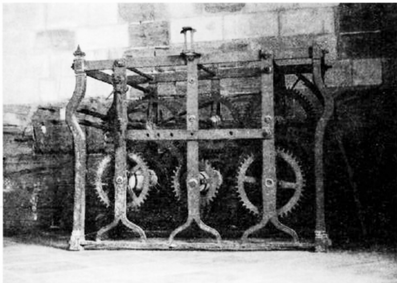
Fig. 1. Relloige de la Seu Vella de Lleida. Situat actualment en una de les capelles del claustre. Indatat
