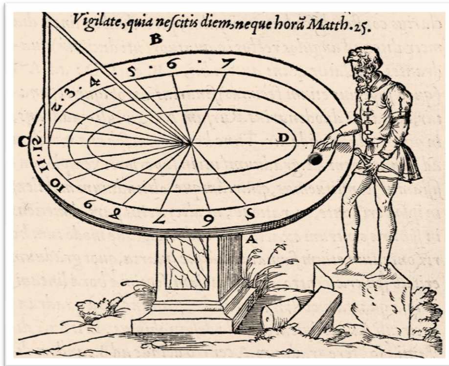
Lib. II 121. Figura horologii horizontalis pro elevatione 42.
