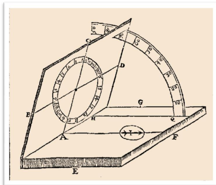
Proposicion XIII. Hazer un reloj equinocial universal.
