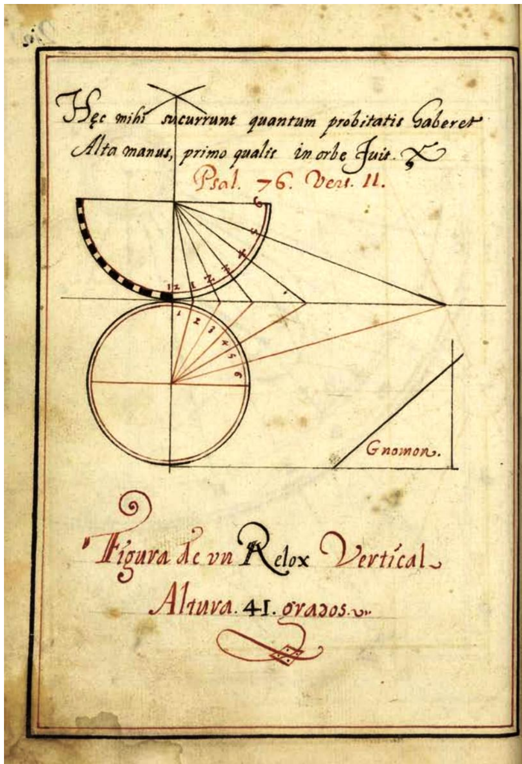
• BNE. Mss/9041. Figura de un Relox Vertical.
